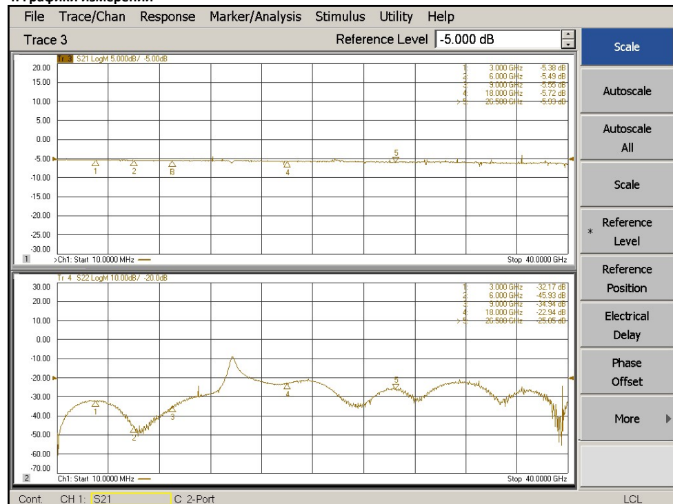
Графики для АЧХ при отсчётном уровне равном -5 дБ и -20 дБ
