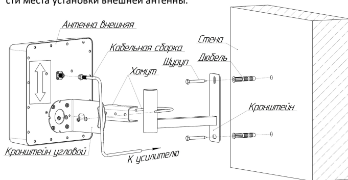
Схема 1 – Монтаж антенны на кронштейн КН-200
