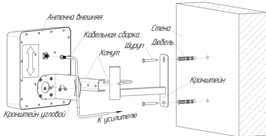
Схема 1 – Монтаж антенны на кронштейн КН-200
