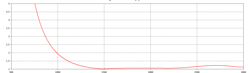
КСВ антенны в рабочем диапазоне частот
