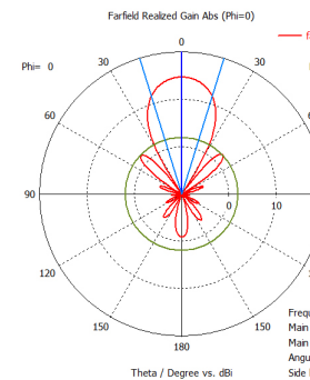
Диаграмма направленности Н-плоскость
