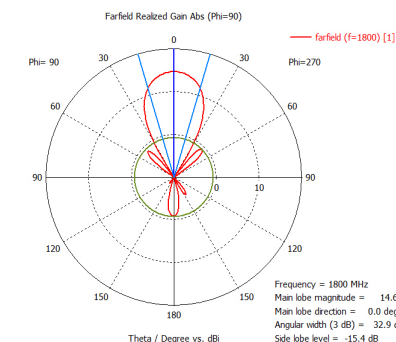
Диаграмма направленности Е-плоскость
