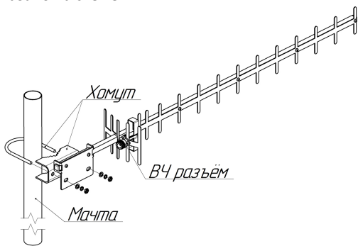
Схема 1 – Монтаж антенны на мачте
