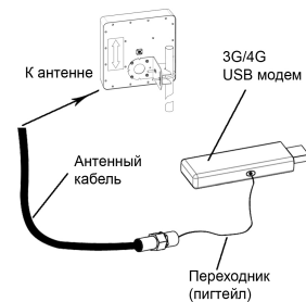
Схема 1 – Подключение USB модема к антенне
