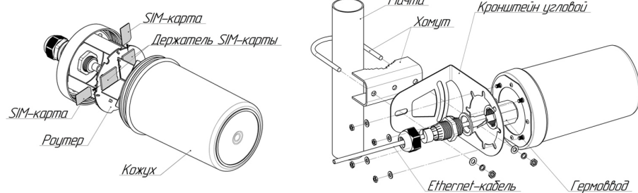
Схема 1 – Сборка роутера с угловым кронштейном и хомутом для монтажа на мачту
