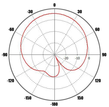
1800 МГц в горизонтальной плоскости
