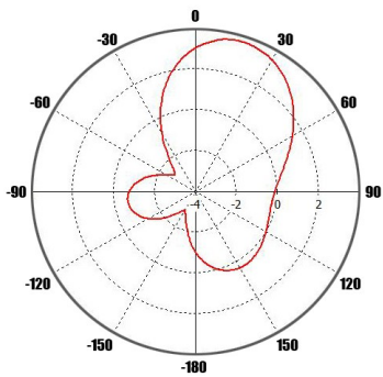
900 МГц в горизонтальной плоскости
