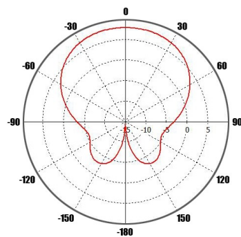
2100 МГц в вертикальной плоскости
