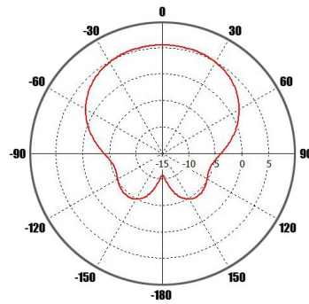
1800 МГц в вертикальной плоскости
