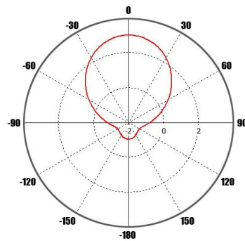
900 МГц в вертикальной плоскости
