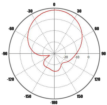
2100 МГц в горизонтальной плоскости
